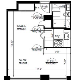
LOGEMENT 101: Superficie 391 sq.ft. ÉCHELLE: 3/16"=1'-0"
