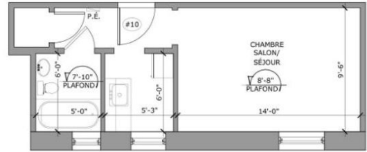
LOGEMENT #10: Superficie 288 sq.ft. ÉCHELLE: 3/16"=1'-0"
